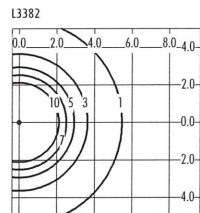
Lyspunkthøjde 1,8m 80W HME (konv.); opal kuppel
