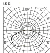
L3383 1 deling = 25 cd/1000 lm \eta_{\text{e}}: 59\% 26W TC-T (konv.); klar kuppel
