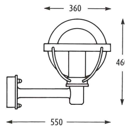
Lyspunkthøjde 1,8m 80W HME (konv.); opal kuppel
