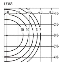
Lyspunkthøjde 1,8m 26W TC-T (konv.); klar kuppel
